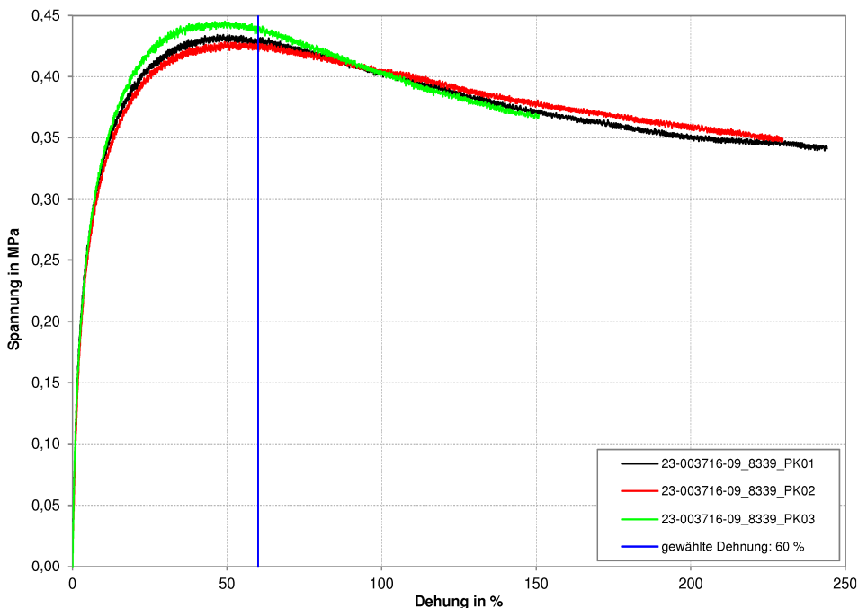
Dehnung bis zum Bruch bei -20 °C, Probekörper 1, 2 und 3
